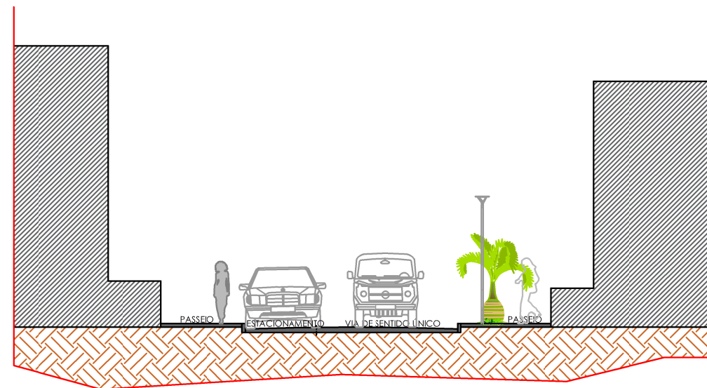
PERFIL XZ
